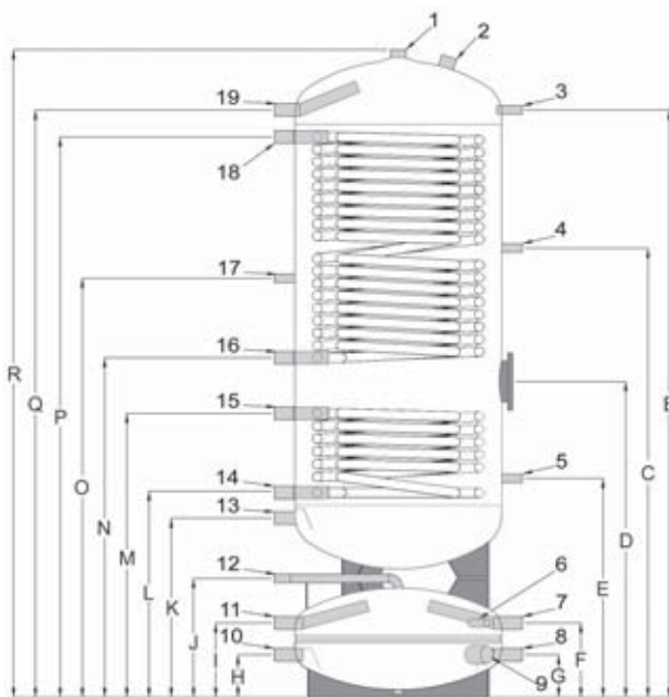
Rozmerový výkres sa vzťahuje k modelu UBHY 500 DC
