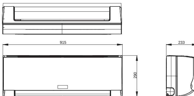
Inštalačná šablóna IQWH20-30
