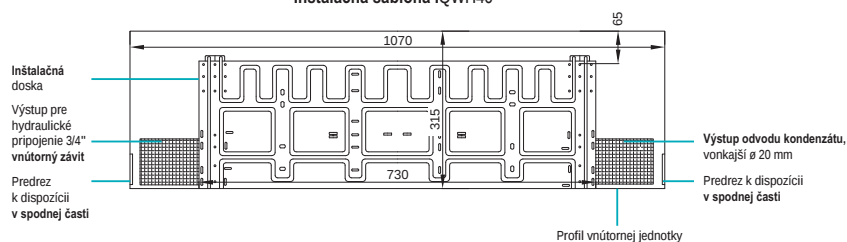
Inštalačná šablóna IQWH40
