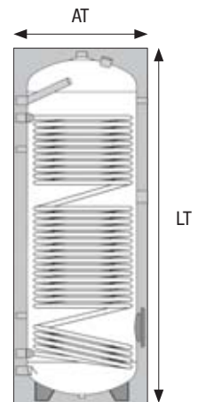
Rozmer s izoláciou
