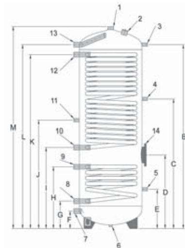
Rozmerový výkres sa vzťahuje k modelu UBHP 300 DC
