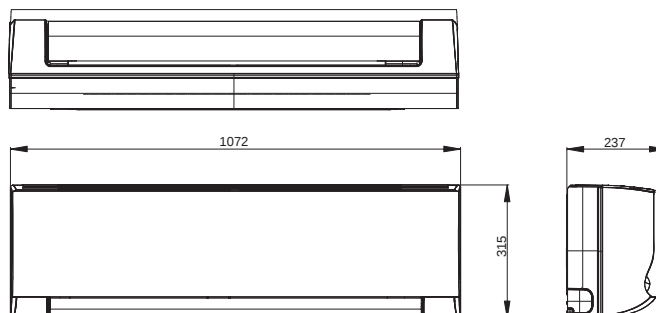
Inštalačná šablóna IQWH40
