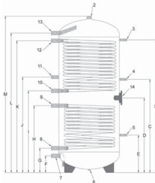
Rozmerový výkres sa vzťahuje k modelu UBHP 1000 DC
