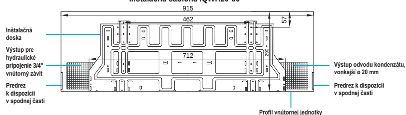
Inštalačná šablóna IQWH20-30
